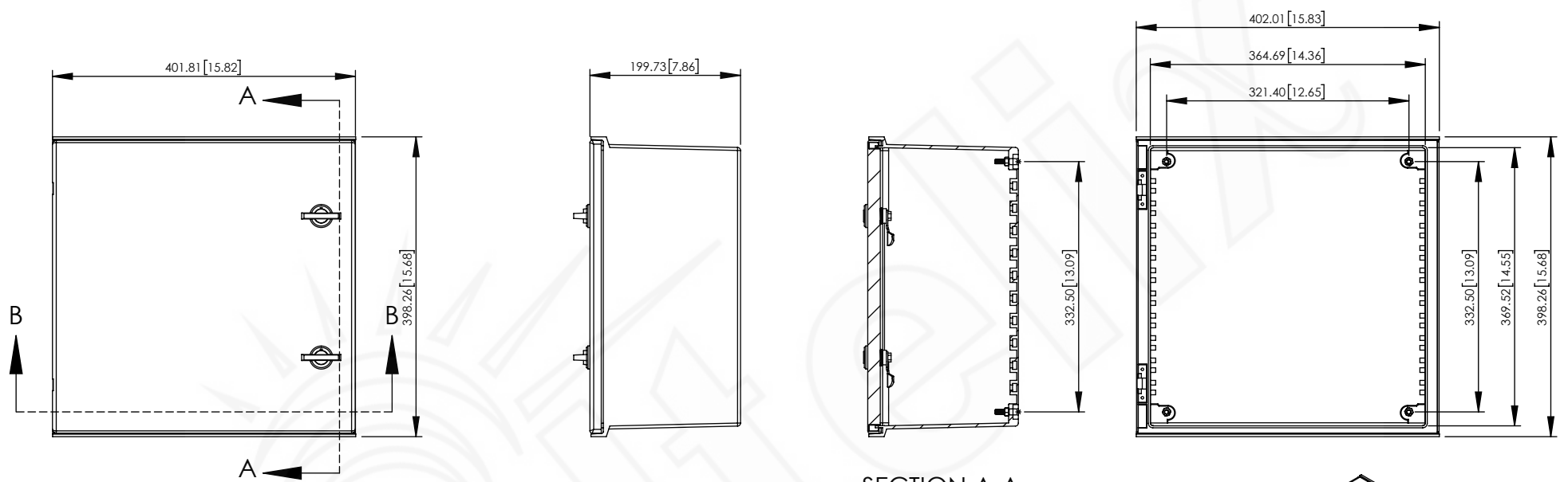
SECTION A-A
